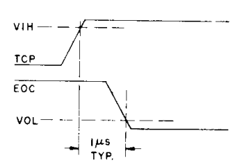
Fig.19 EOC TURN-OFF
